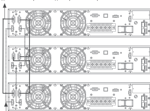
Рисунок 3. Схема подключения параллельного резервирования 3х ИБП
