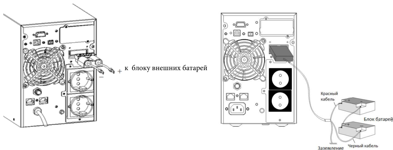
Рис. 5 Подключение батарей к ИБП ONLINE PLUS
