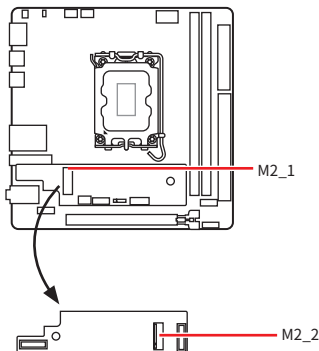
Вид сверху на материнскую плату
