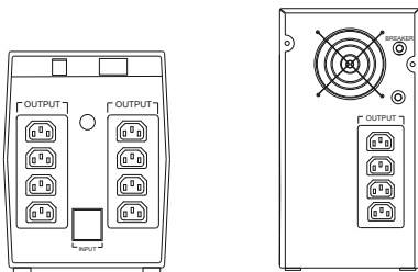
Рисунок 5 – Задняя панель ИБП без коммуникационного порта или с портом USB (опционально) и разъемами С13
