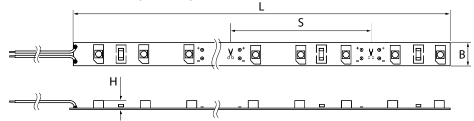
Рис. 1 Лента светодиодная
